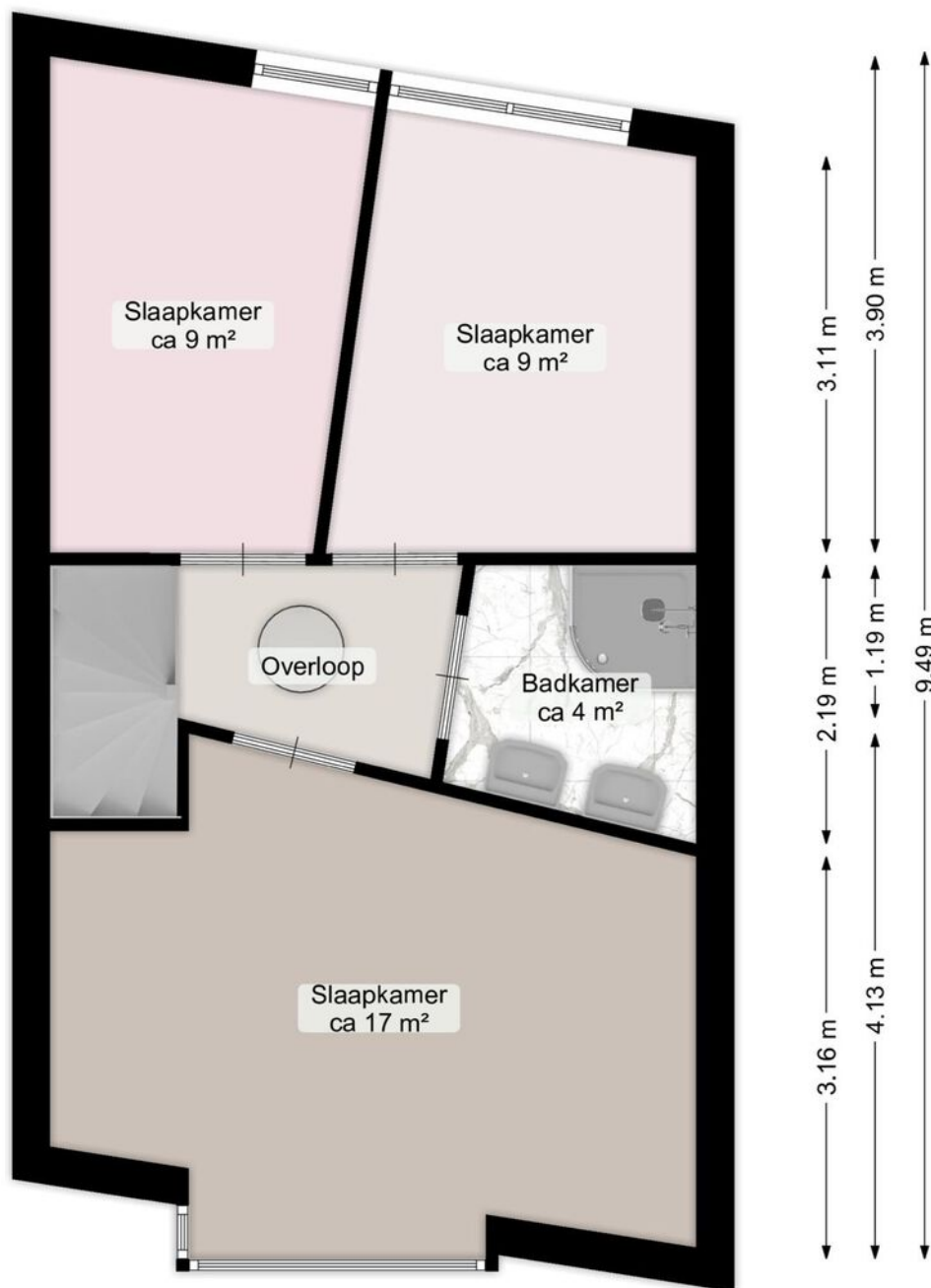
Eerste verdieping
