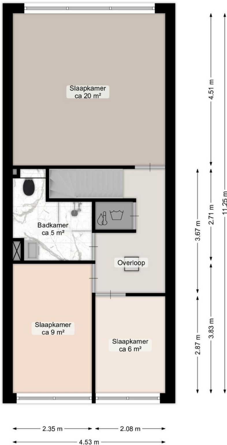
Tweede verdieping
