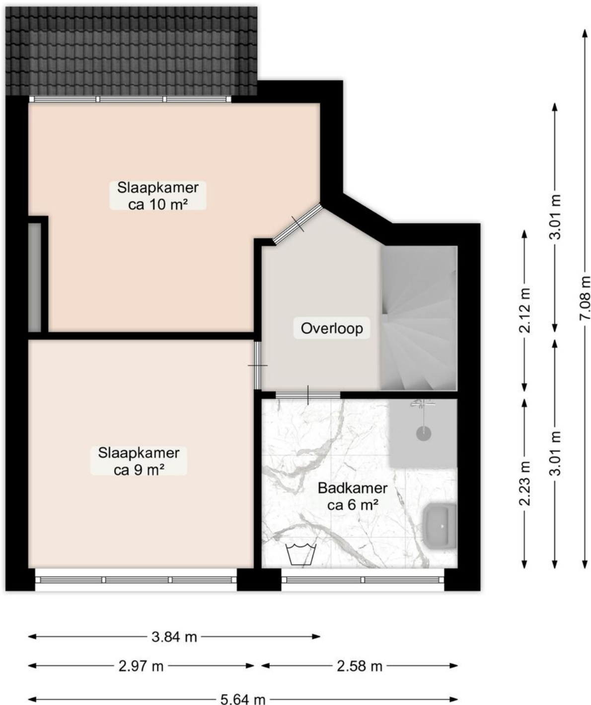
Tweede verdieping
